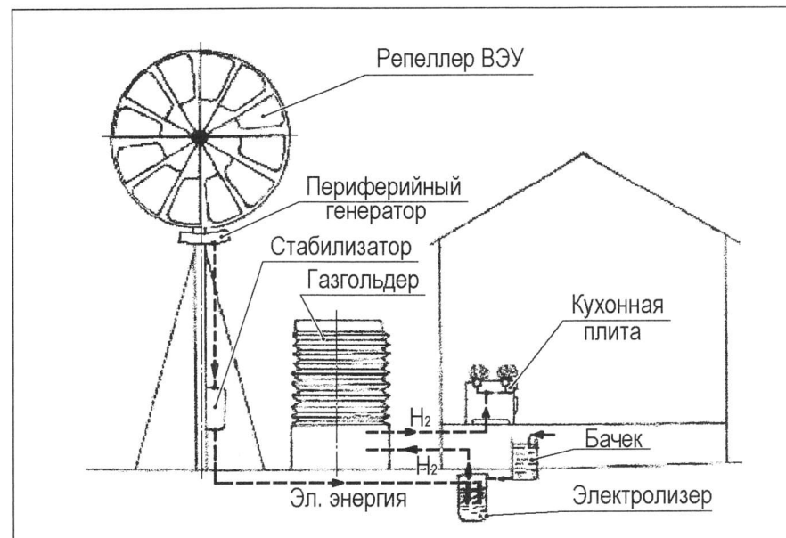
Рис. 1. Схема ветроплавильной установки с накоплением горючего в газгольдере или баллонах высокого давления.
