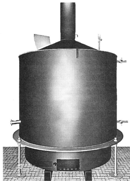
Теплоагрегат «ТУБ» Сорокин-Кучин.
