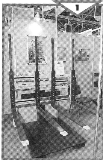
Такие вилы можно сдвигать и раздвигать, перевозить на них несколько поддонов.
